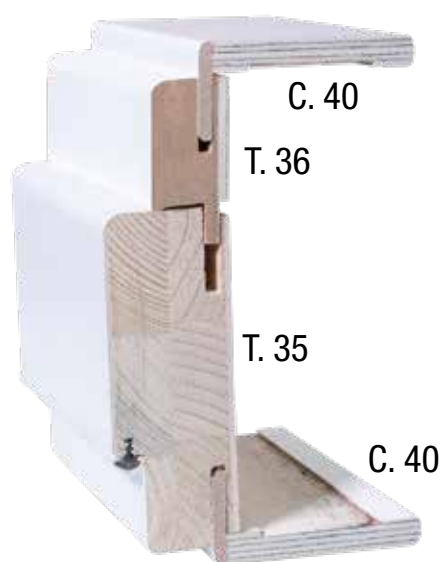
Telaio con allargamento
