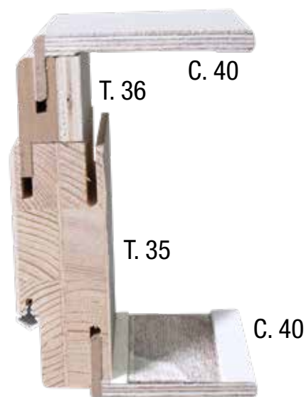
Telaio con allargamento + cornice PLUS
