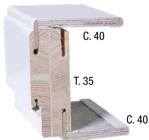
Telaio standard + cornice PLUS
